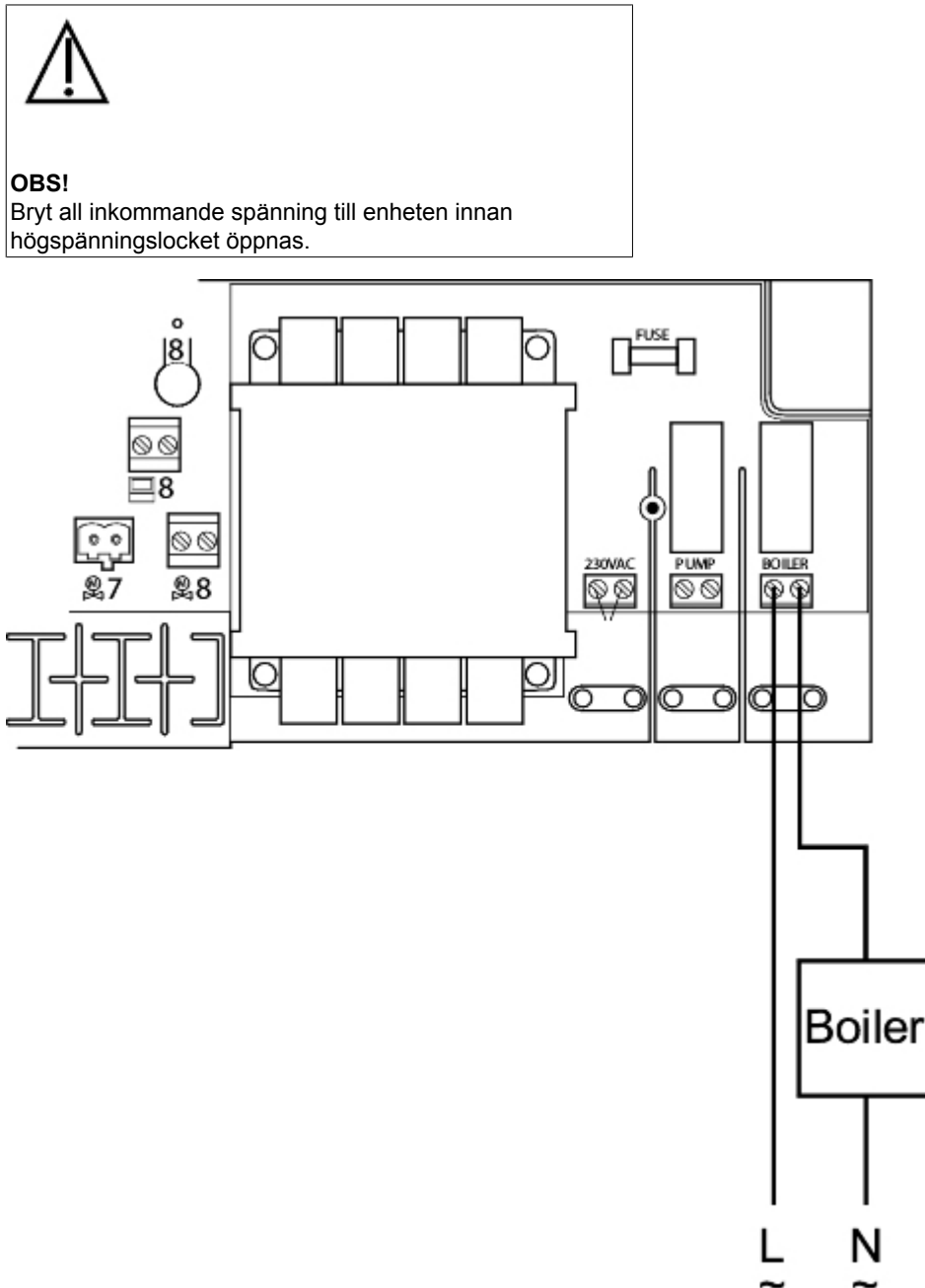
Kopplingsschema för inkoppling av värmekälla till mottagarenhet ICS 8.
